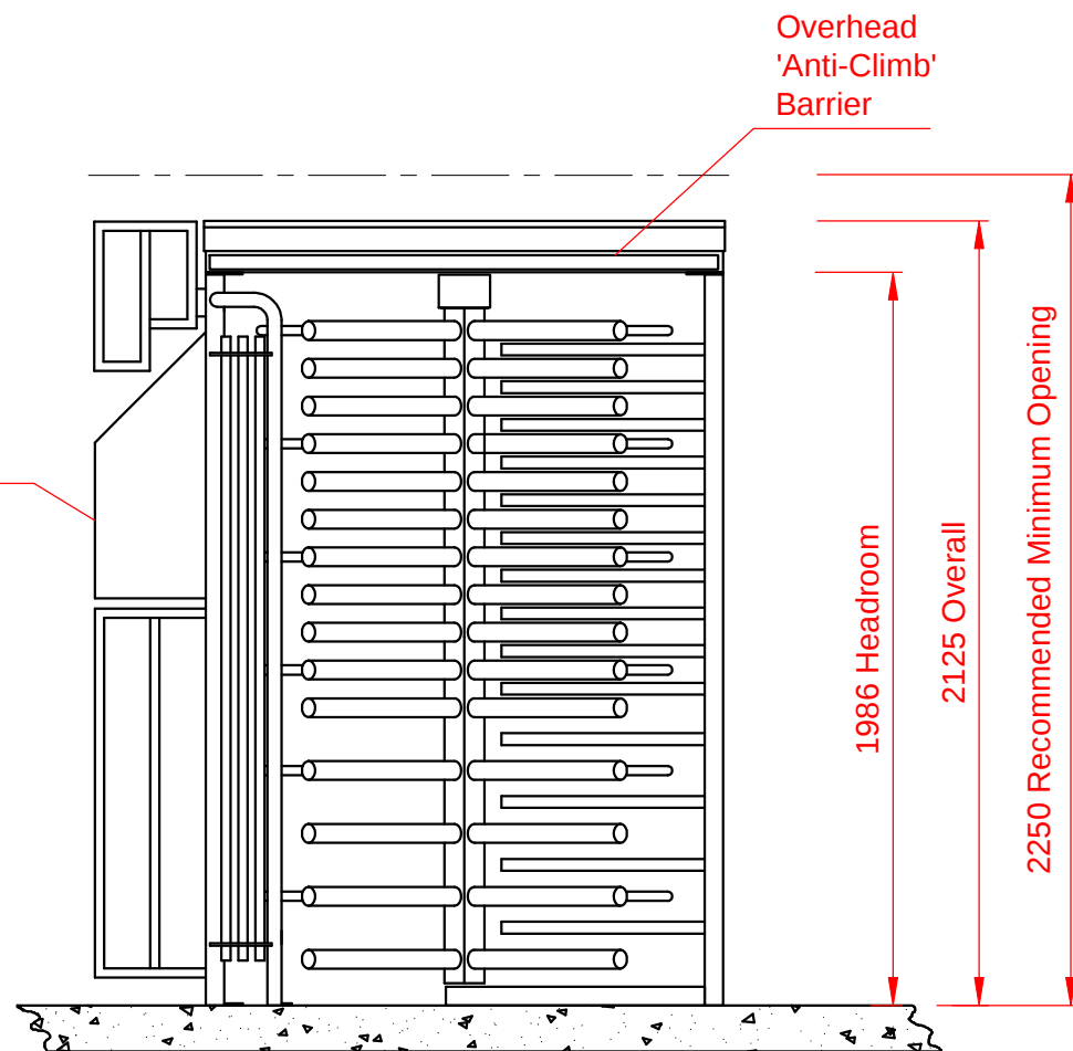
ELEVATION
