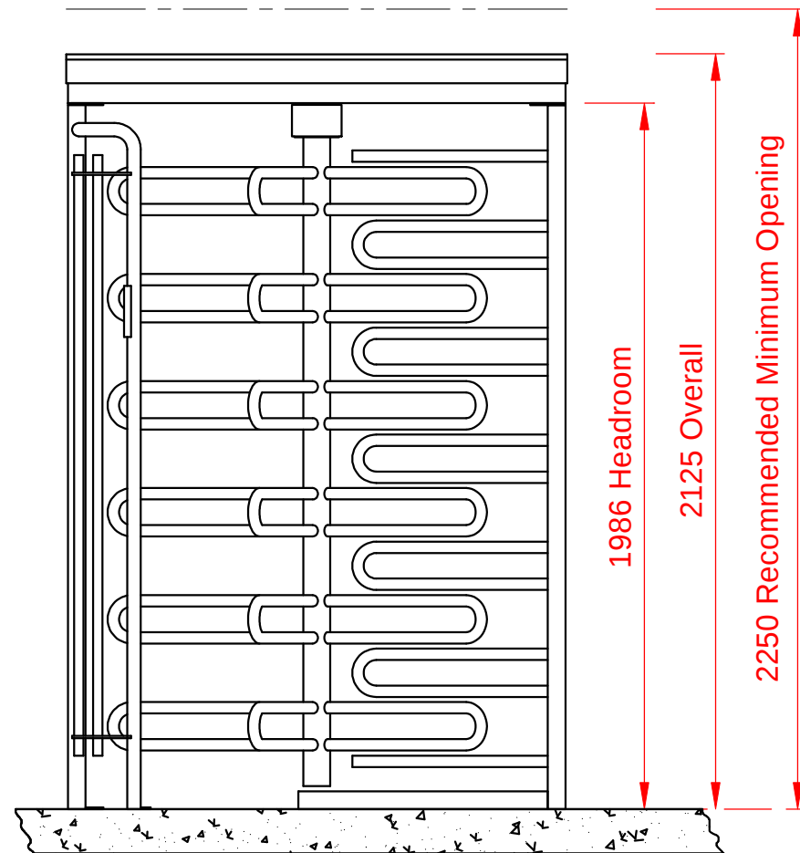
ELEVATION
